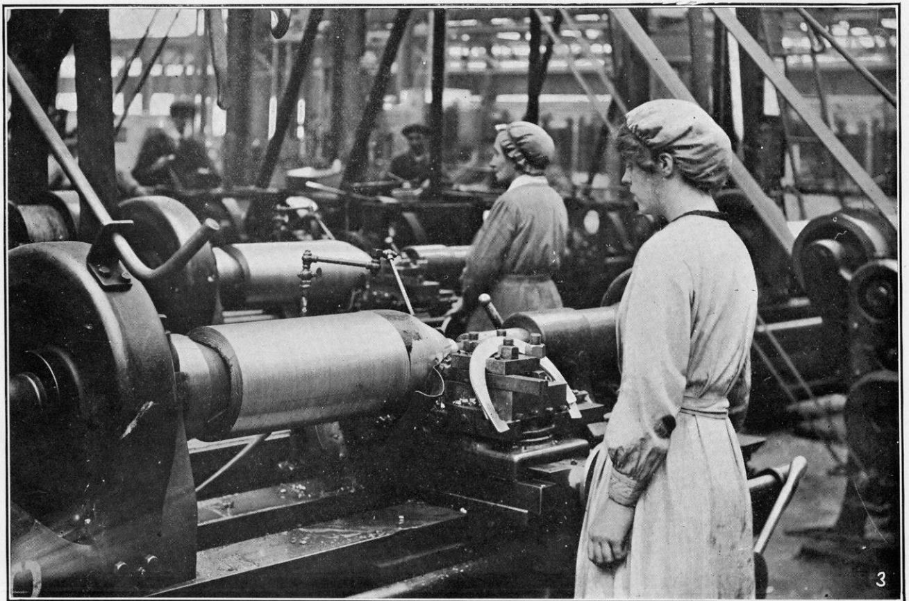
Kvinder i Arbejde med 9.2 Tommers Granater med stor Sprængvirkning.—1. Tilpasning og Tilskruning af Næsespidsen paa en Granat. 2. En Granat undersøges. 3. Raadrejning af en Granat.
