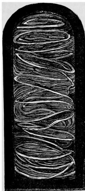
FIG. 2.—Striæ above critical point
