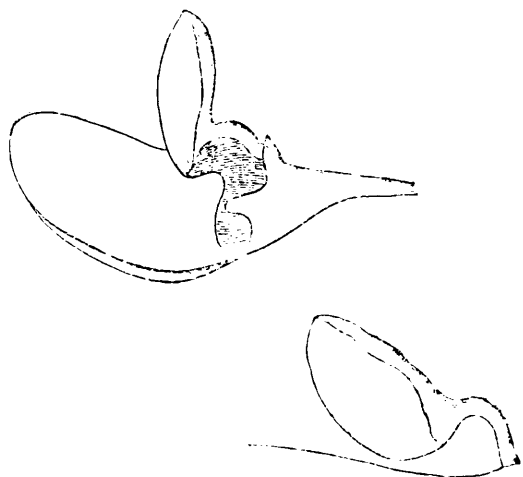
FIG. 1.— Coronilla varia .
