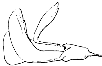
FIG. 2.— Coronilla emerus .
