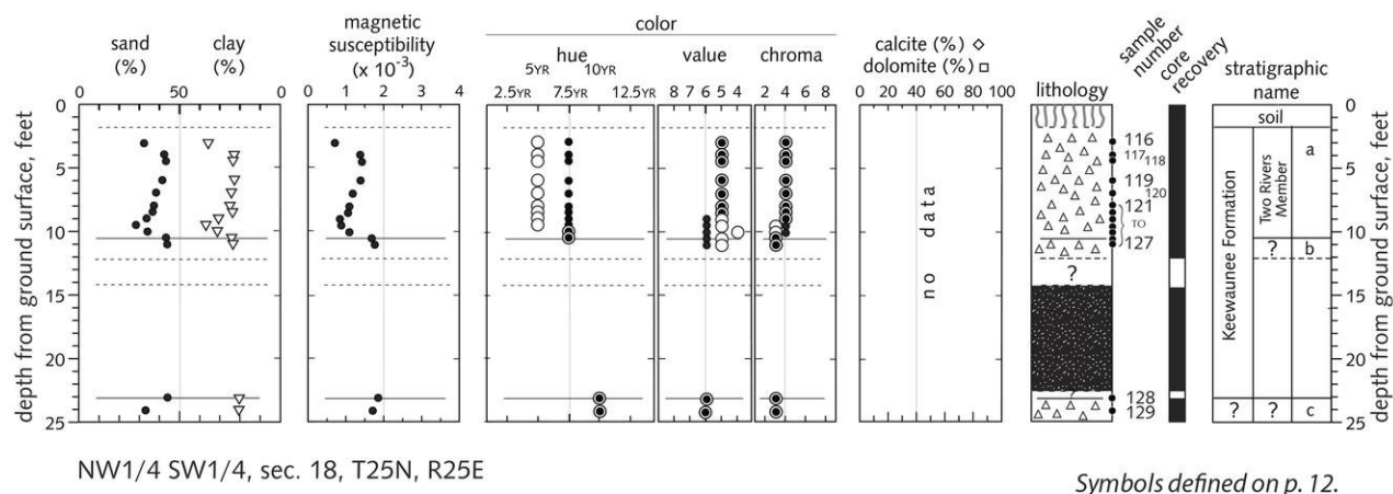
Figure 10b. Sample log for drill hole KL.
