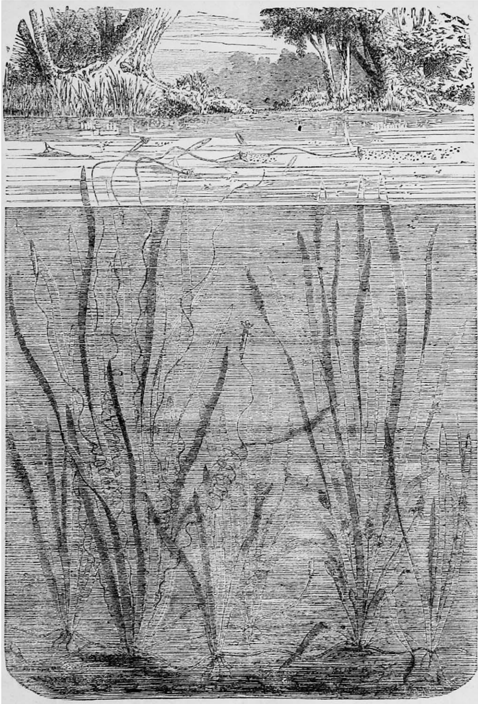
FIG. 2.— Vallisneria spiralis
