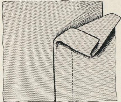
Fig. 257. Welt Seam
