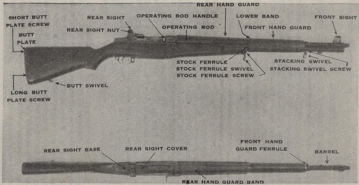
FIGURE 7.—U. S. rifle, caliber .30, M1.
